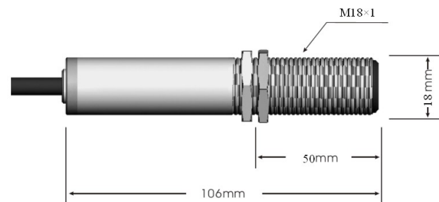
红外线测温仪外型尺寸
